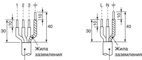
Соединительный кабель
